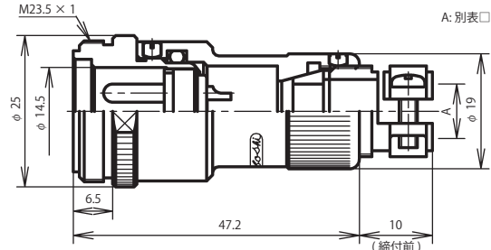
NWPC-16 ■ -Ad □ -CH
