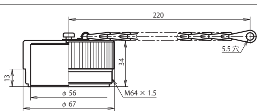
プラグキャップ：NWPC-60-PCa
