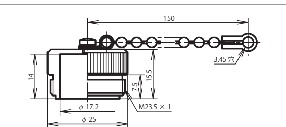
プラグキャップ：NWPC-16-PCa
