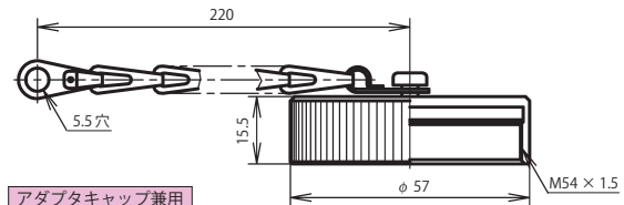
レセプタクルキャップ：NWPC-50-RCa
