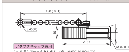
プラグキャップ：NWPC-30-PCa
