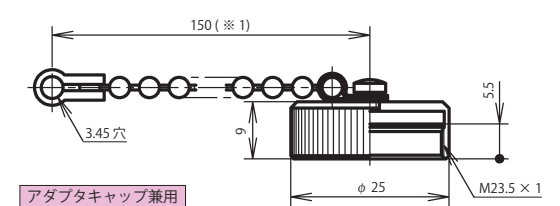
プラグキャップ：NWPC-16-PCa
